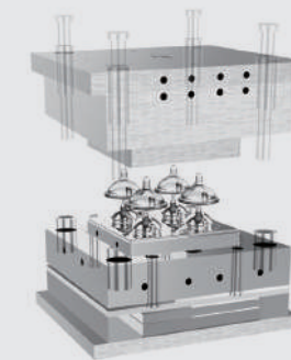
LSR 젓꼭지 금형모델링
