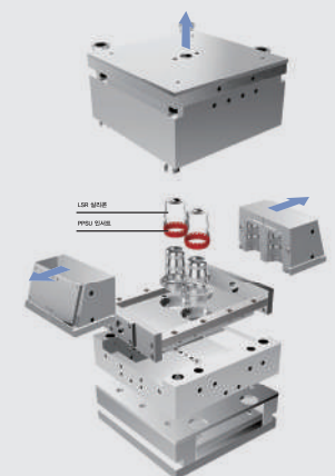
LSR 젓병 금형모델링
