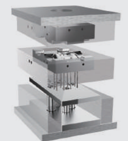
의료용 경추신경기 금형모델링
